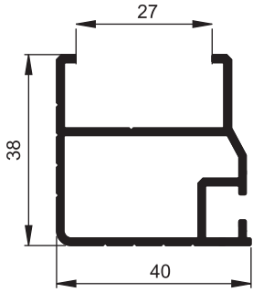
2117 K 0.708 kg/m Kola Dolap Profili
