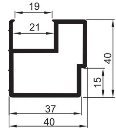
2117 D 0.955 kg/m Kola Dolap Profili ( Çıtasız )
