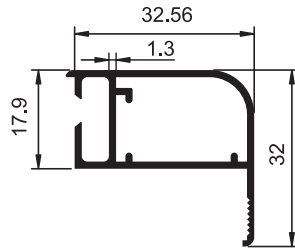
2117 U 0.437 kg/m Kola Dolap Profili
